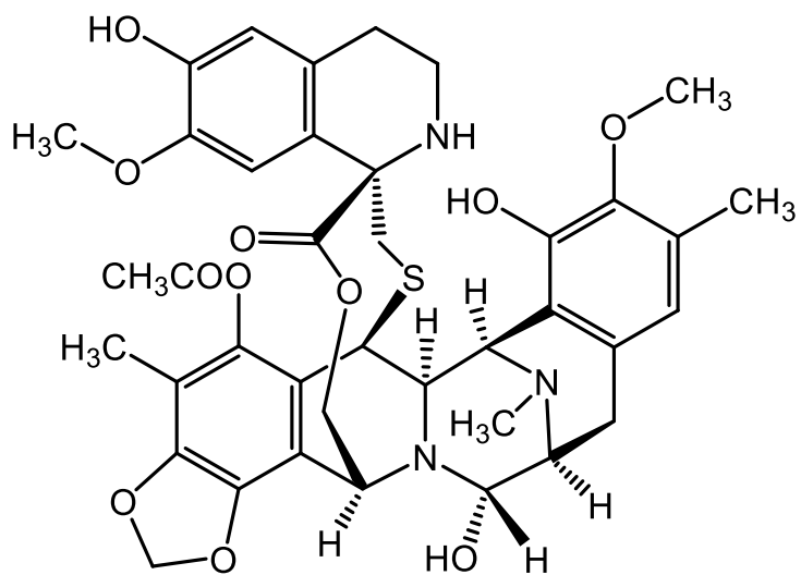
Ecteinascidin 743
