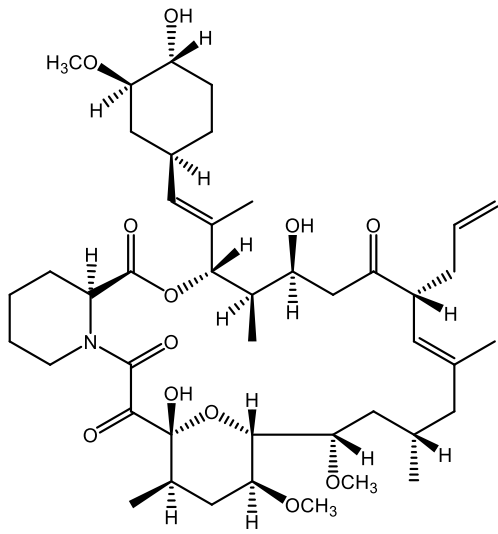
Tacrolimus (FK506)
