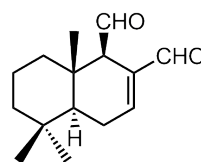
Polygodial
